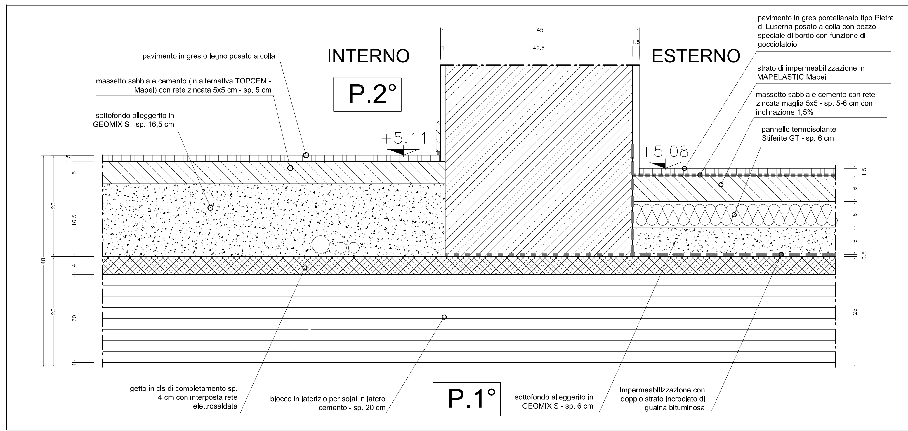
STRATRIGRAFIA SOLAIO TERRAZZO - scala 1:5
