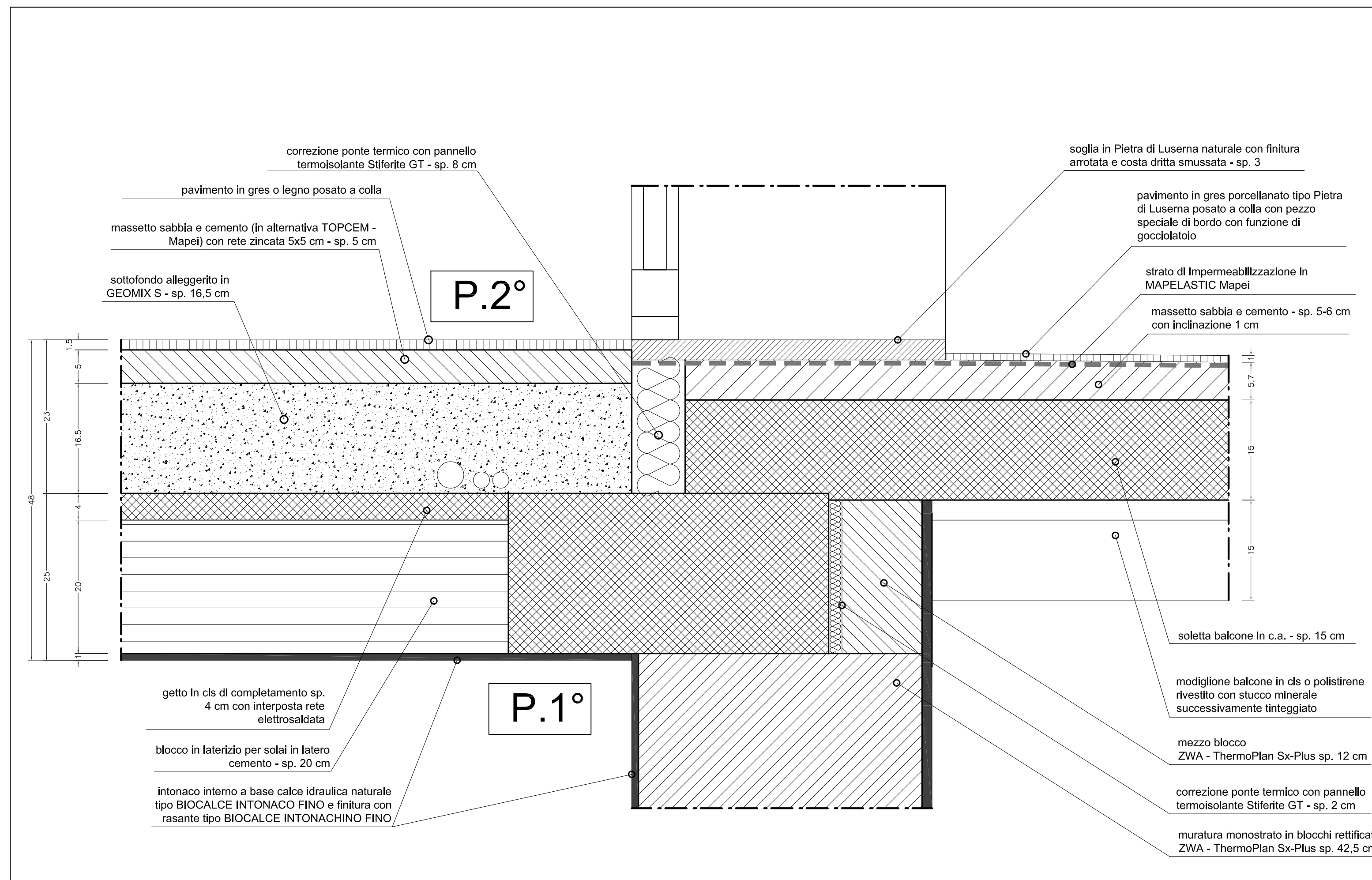
STRATRIGRAFIA SOLAIO INTERPIANO - scala 1:5
