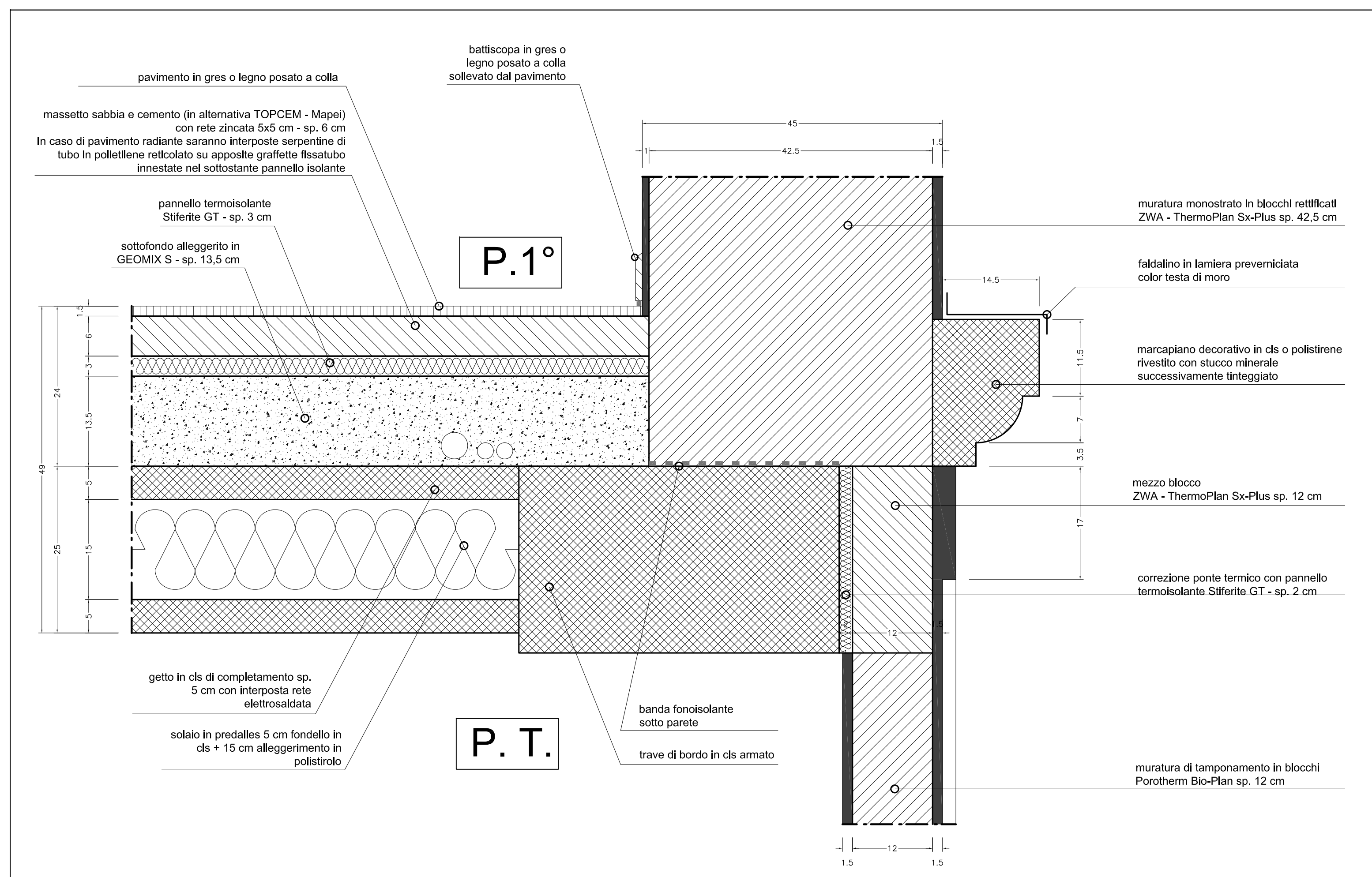
STRATRIGRAFIA PRIMO SOLAIO - scala 1:5 (medesima stratigrafia in caso di pavimento radiante a qualunque piano)
