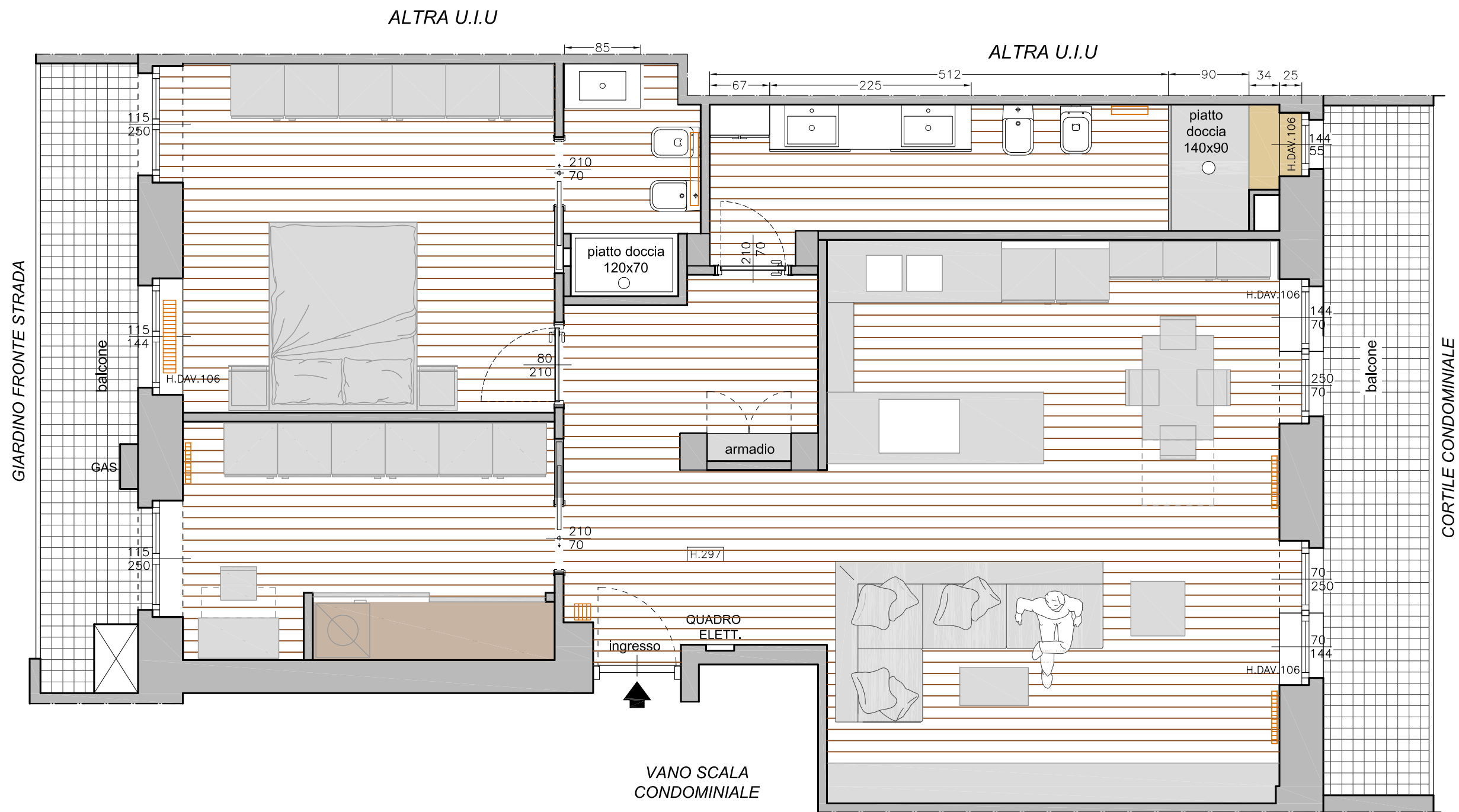
PROGETTO CON ARREDO - PIANTA PIANO PRIMO - SCALA 1:50
